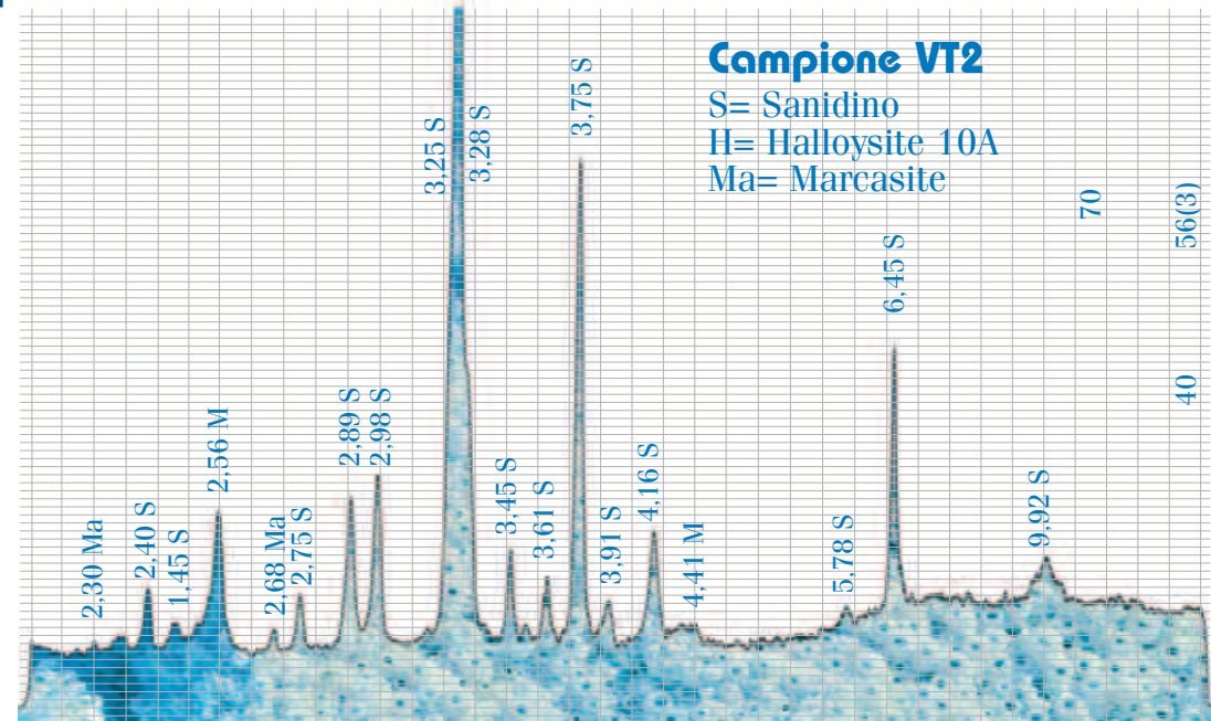
[1] Esempio di analisi diffrattometrica 🇬🇧 Example of a Diffractometric analysis 🇩🇪 Beispiel einer diffraktometrischen Analyse
